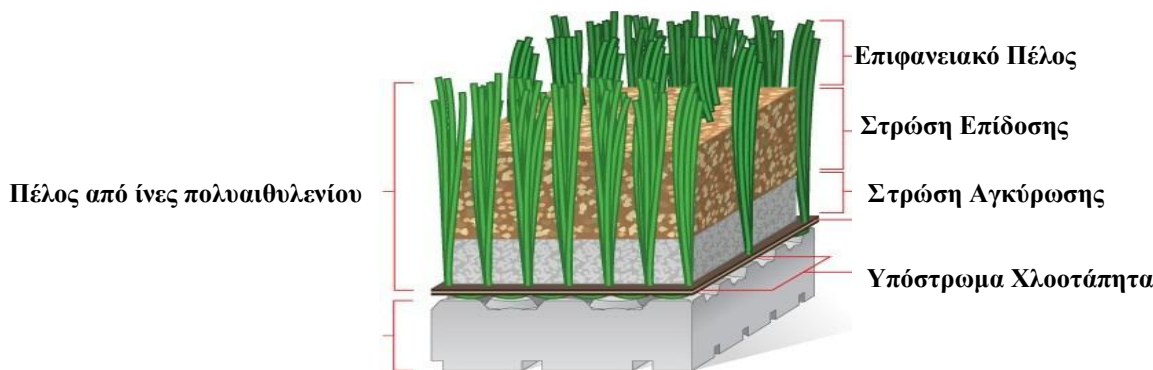
Σχ. 1. Τυπική τομή Ποδοσφαιρικού τάπητα τύπου έξι (6) πίνακα A.6 EN 15330-1:2013-12
